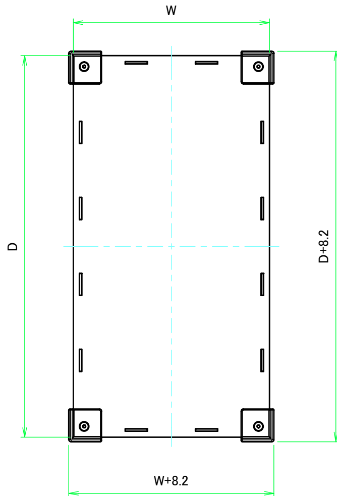
上カバー / Top cover
