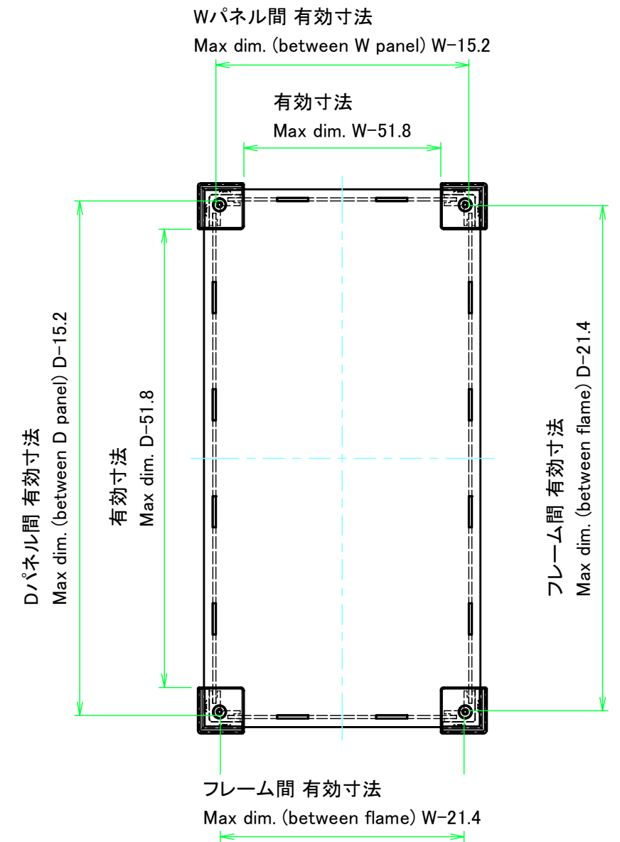
下カバー / Bottom cover
